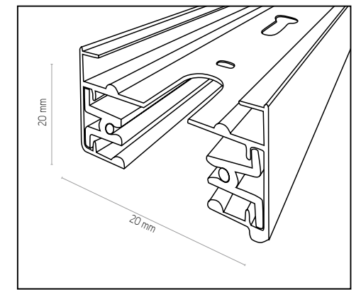
PRZEKRÓJ LISTWY PROWADZĄCEJ
